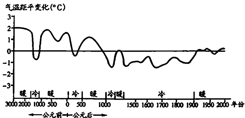
(5000年来我国气温距平变化图)(图8)
