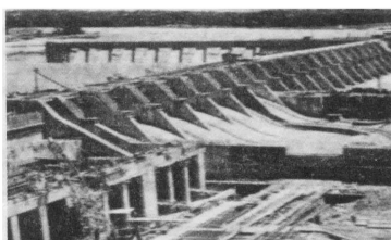
危机期间完成的田纳西水利工程
